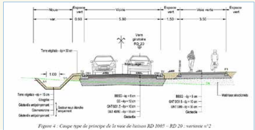
Figure 4 : Coupe type de principe de la voie de liaison RD 1005 - RD 20 : variante n°2
